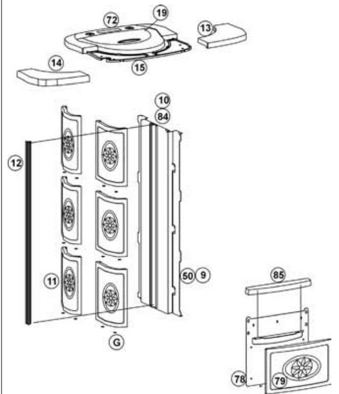
G: Gummiprofile zur Einfügung zwischen den seitlichen Keramikelementen
